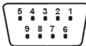
PC COM1 9 芯针座
