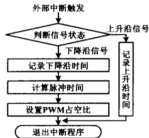
图 6 调速信号检测流程图
