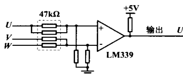
图 4 反电势检测电路
