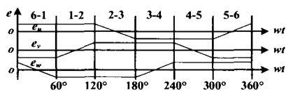
图 2 反电势过零法的工作原理
