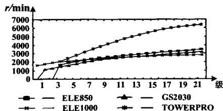
图 9 电机驱动测试结果
