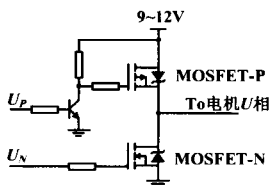
图 5 电机驱动电路
