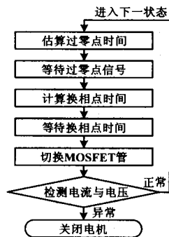
图 7 电机换相控制流程图
