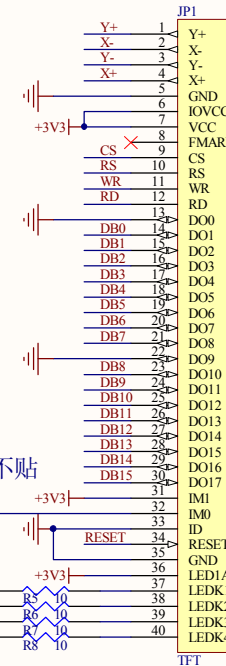
3.0寸 (400 * 20) TFT接口
