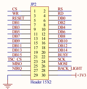
CPU接口
