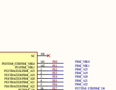
256K * 16 SRAM扩展
