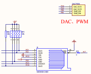
micro SD卡(SDIO模式)
