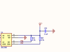
串行EEPROM (1KB)
