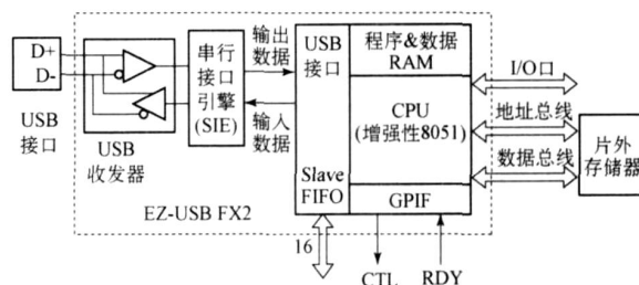
图 2 128脚 FX2框图
