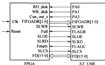
图 1 系统连接框图
