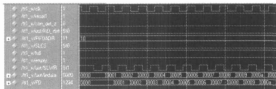
图 5 写数据仿真波形
