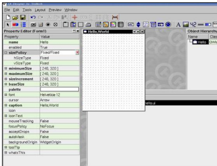
图 12.18 Hello 窗体的属性设置
