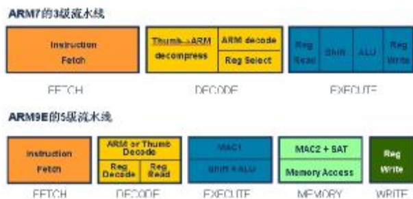
图 4.4 ARM7 与 ARM9 流水线比较
