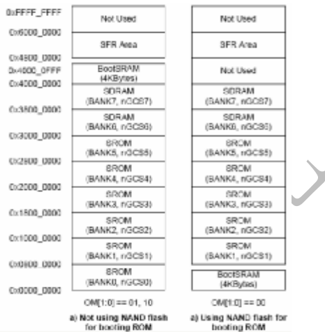
图 4.12 S3C2410 两种启动模式地址映射
