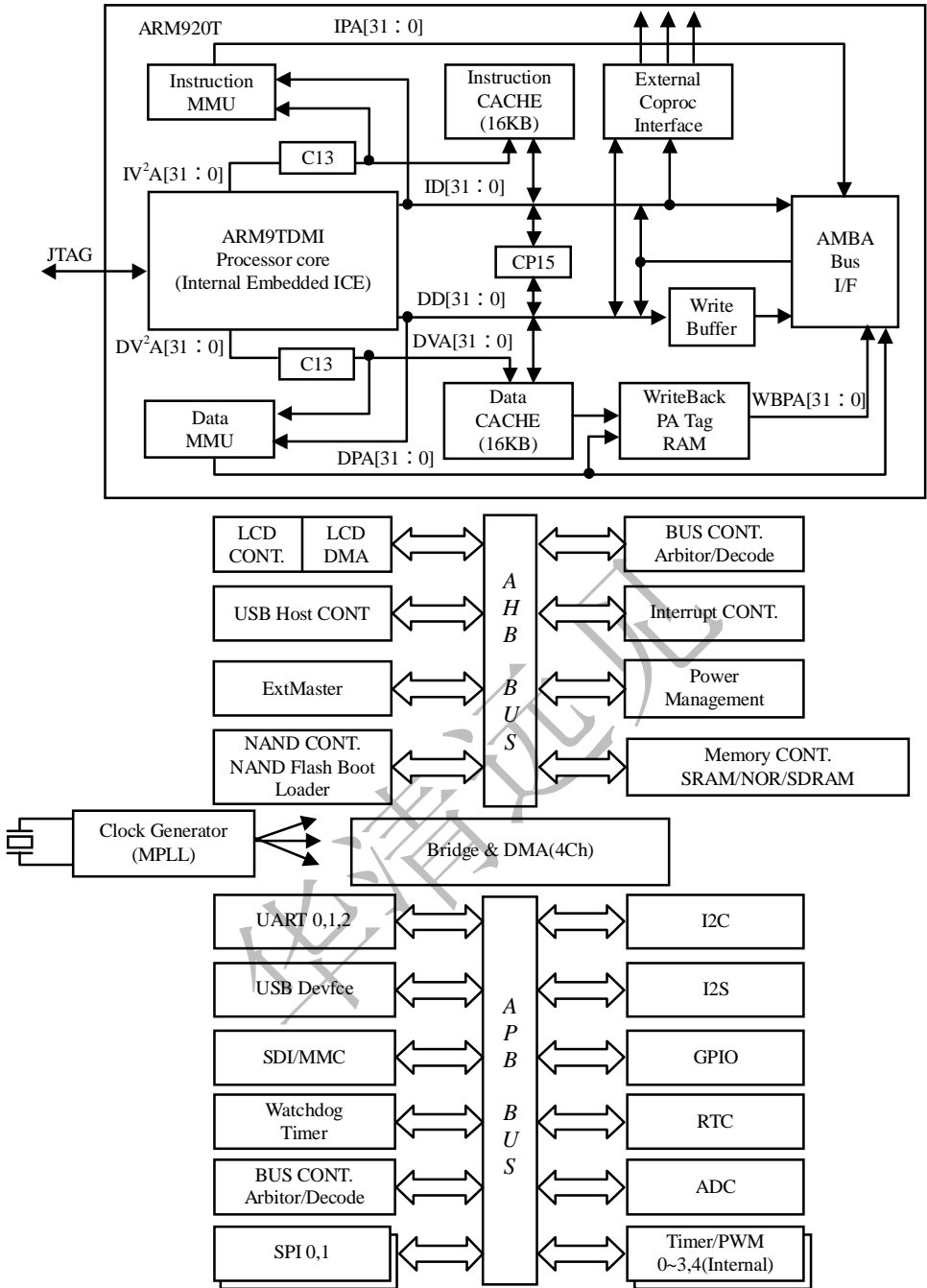
图 4.11 S3C2410X 系统结构图
