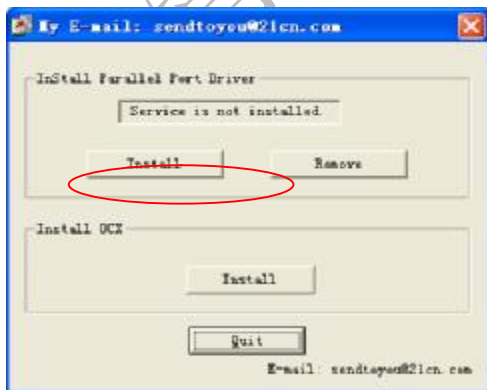
图 4.24 安装 giveio
