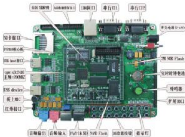
图 4.10 优龙 FS2410 开发板实物图
