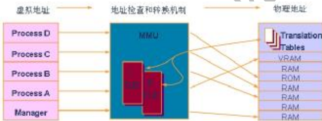
图 4.8 MMU 的实现过程
