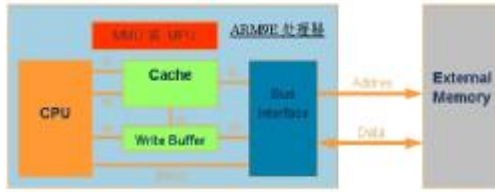
图 4.7 ARM9 的高速缓存和读缓存
