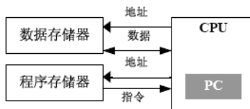
图 4.6 哈佛结构
