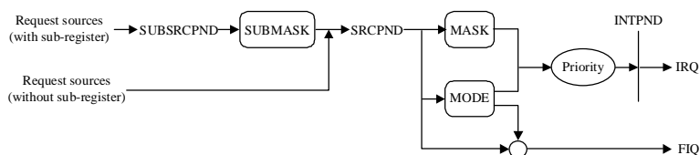
图 4.14 S3C2410X 中断处理流程
