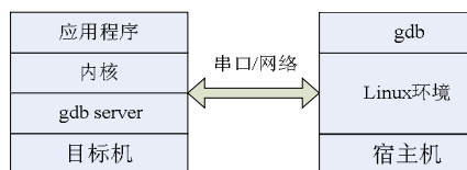
图 4.19 gdb 远程调试原理图
