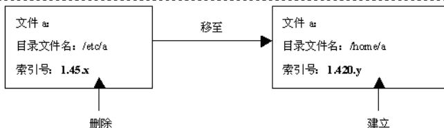
图 1.5 目录文件与索引节点关系
