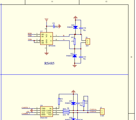
CAN总线
