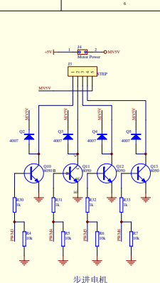
步进电机
