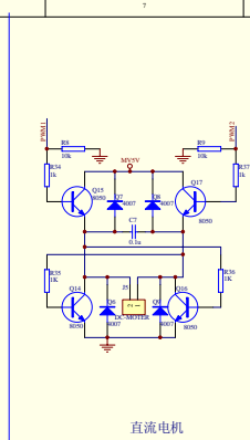
直流电机
