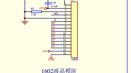
1602液晶模块
