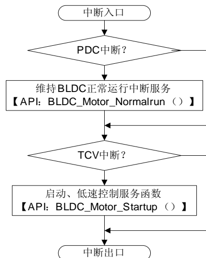
图 5-2 PDC、TCV 中断操作流程
