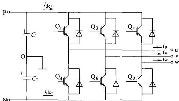
图1 三相逆变器主电路图
