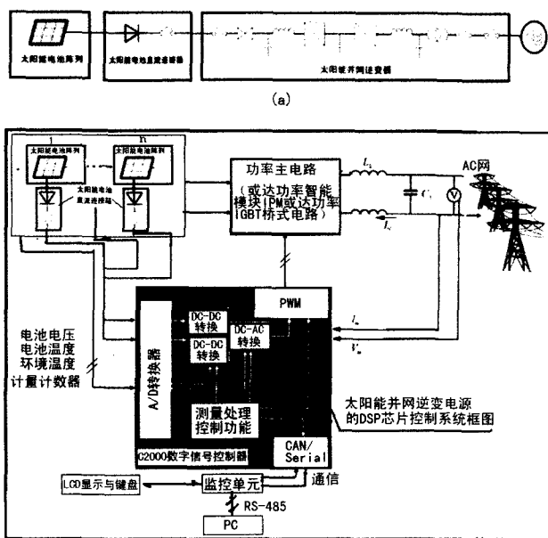
图3 (a) 太阳能并网逆变电源基本设计方案框图; (b) 以TMS320C2000 DSP为控制系统的太阳能并网逆变电源设计方案示意图
