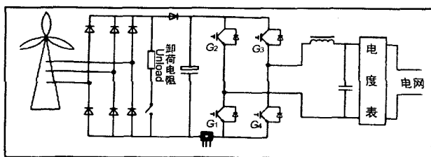
图6 风机并网逆变电源框图
