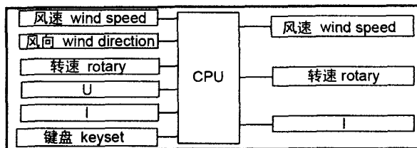
图5 无尾翼风机控制器原理图
