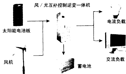
图4 风光互补发电系统组成示意图
