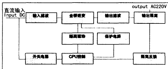
图2 逆变电源基本工作框图
