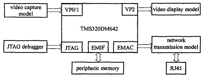
Fig.1 DM642's main function model 图 1 DM642 主要功能模块
