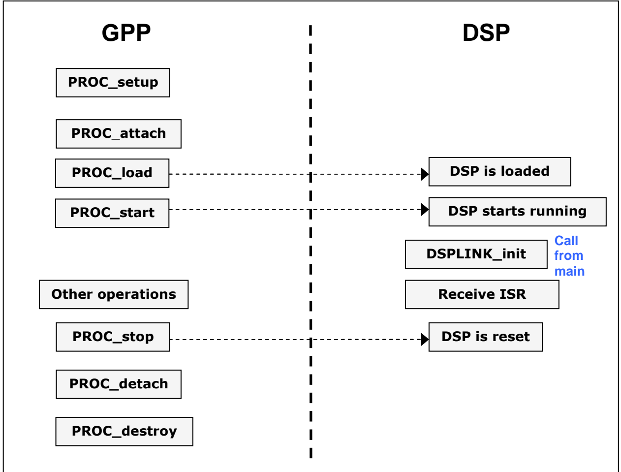
Figure4. NormalBootMode
