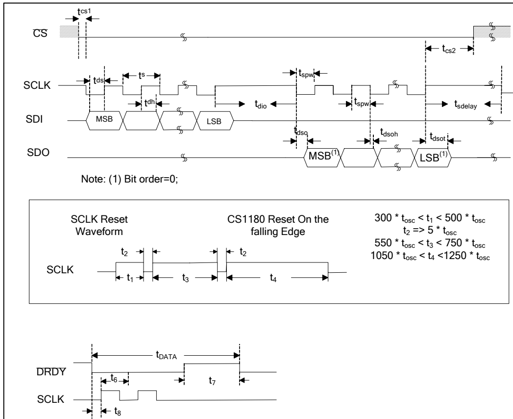
图3 CS1180 时序图
