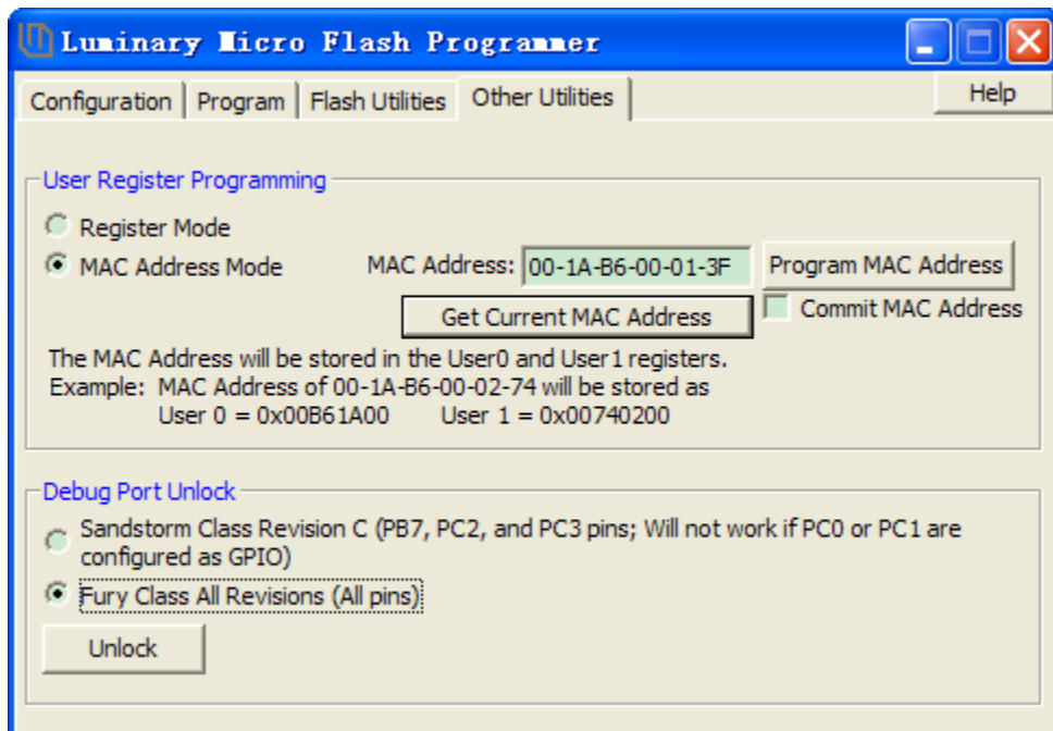
图 3 调试端口解锁
