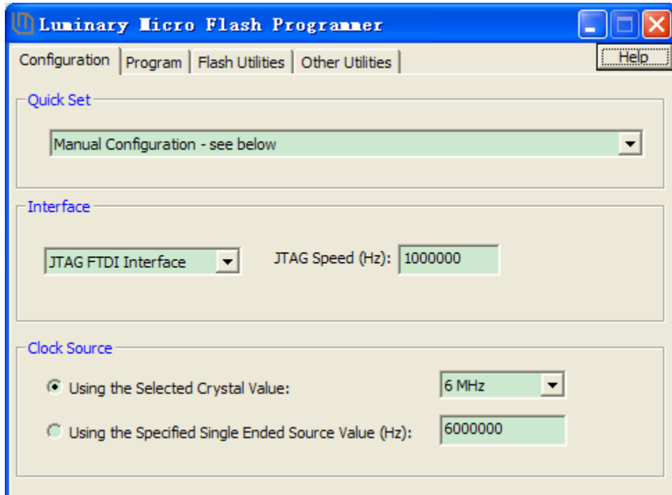
图 2 Flash Programmer 配置选项
