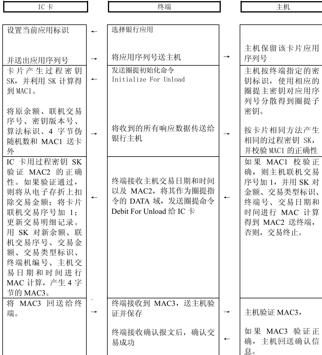
图 7-3 圈提交易流程
