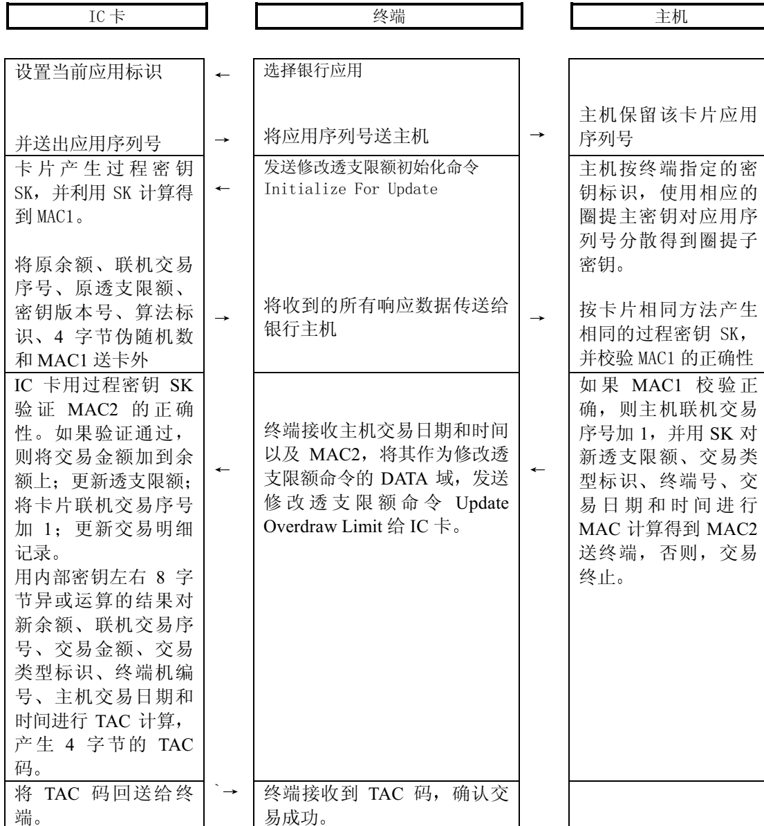
图 7-4 修改透支限额交易流程
