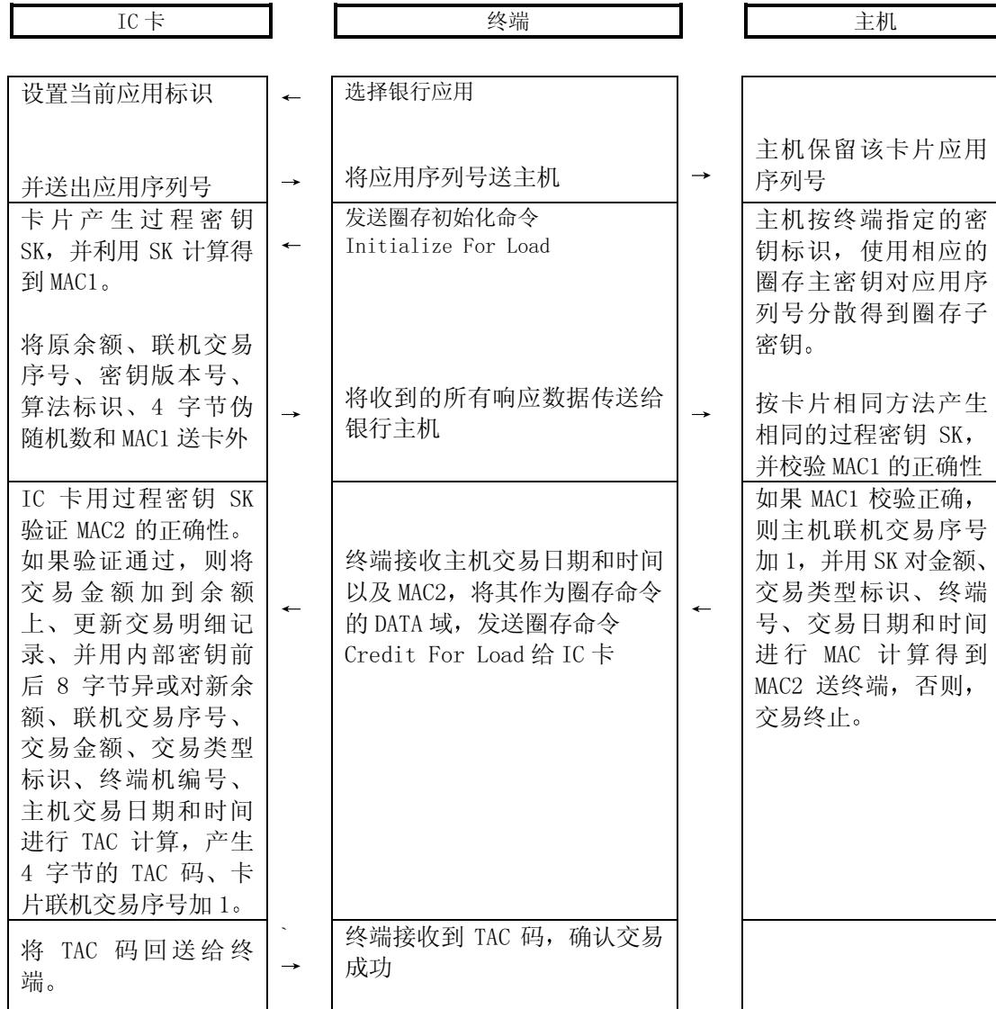
图 7-1 圈存交易流程
