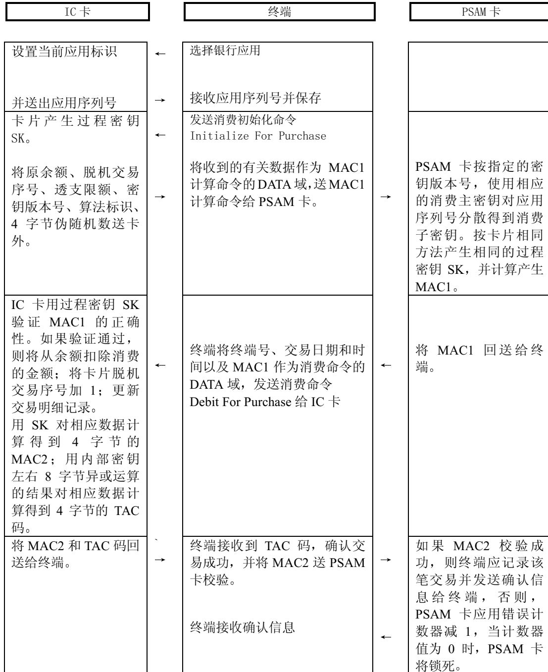
图 7-2 消费交易流程
