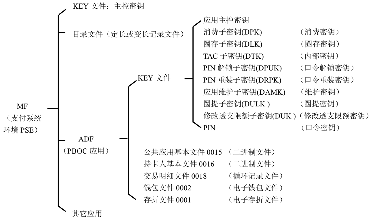
图 3-1 TimeCOS/DI 文件结构举例（简要）
