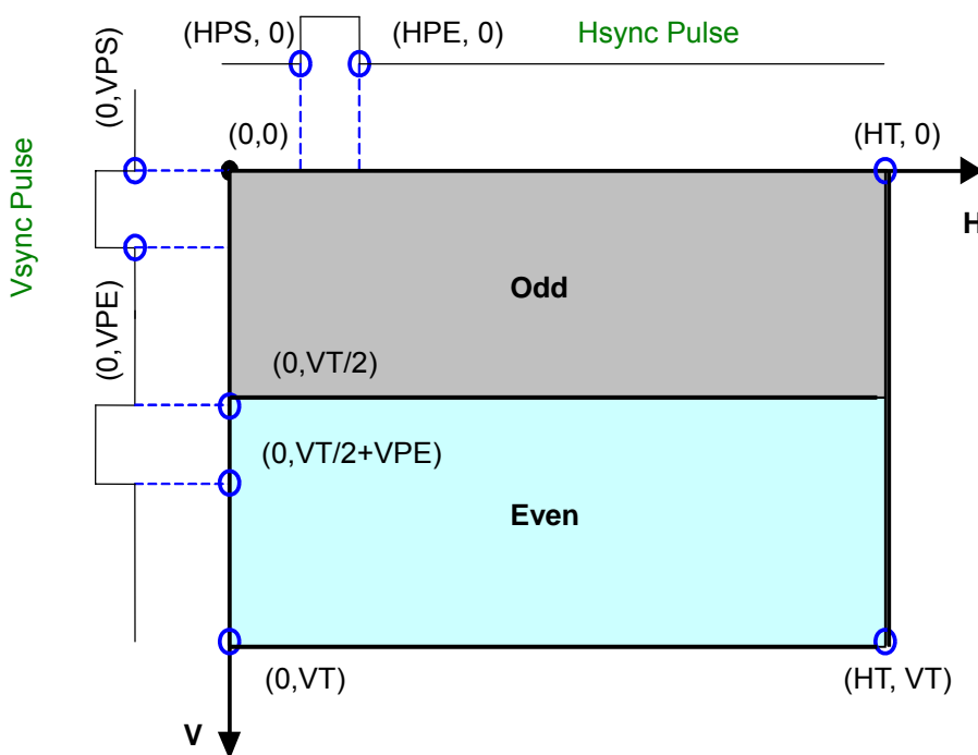
Figure 11-2 TV-Encoder Display Parameters
