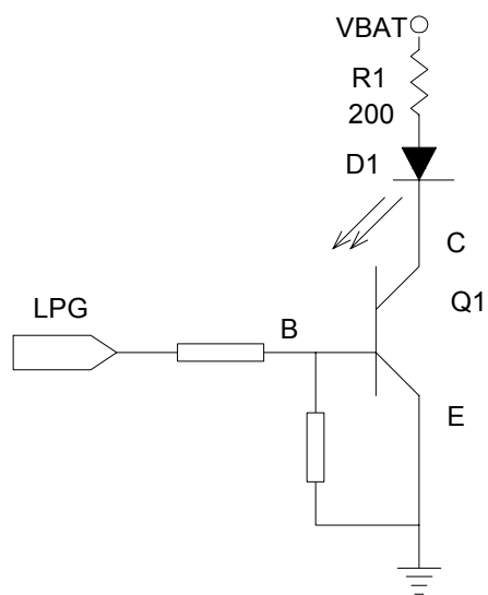
图4-11 LPG 外部电路示意图
