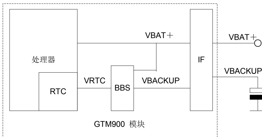
图4-5 RTC Backup 电路示意图
