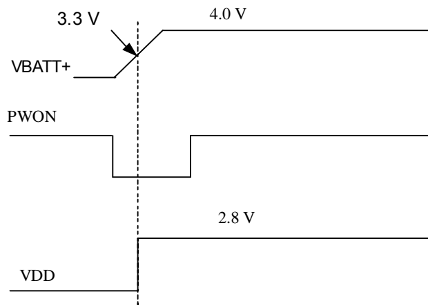
图5-1 VDD 与 PWON 信号的关系
