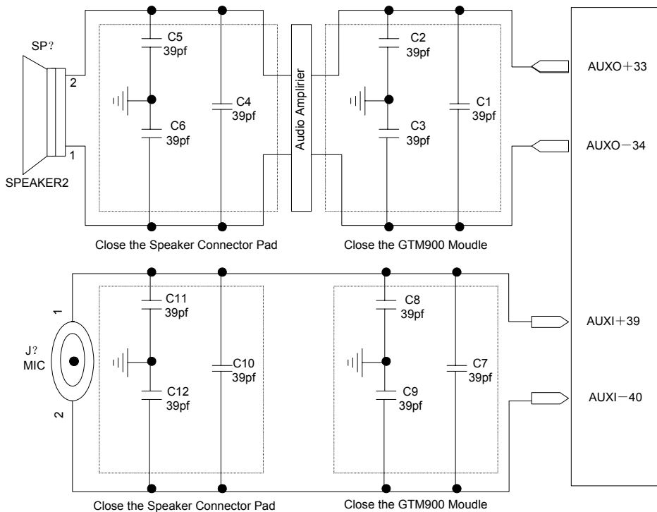
图4-7 第二路音频信号连接示意图
