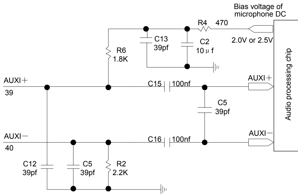
图4-9 第二路音频输入通道的电路示意图
