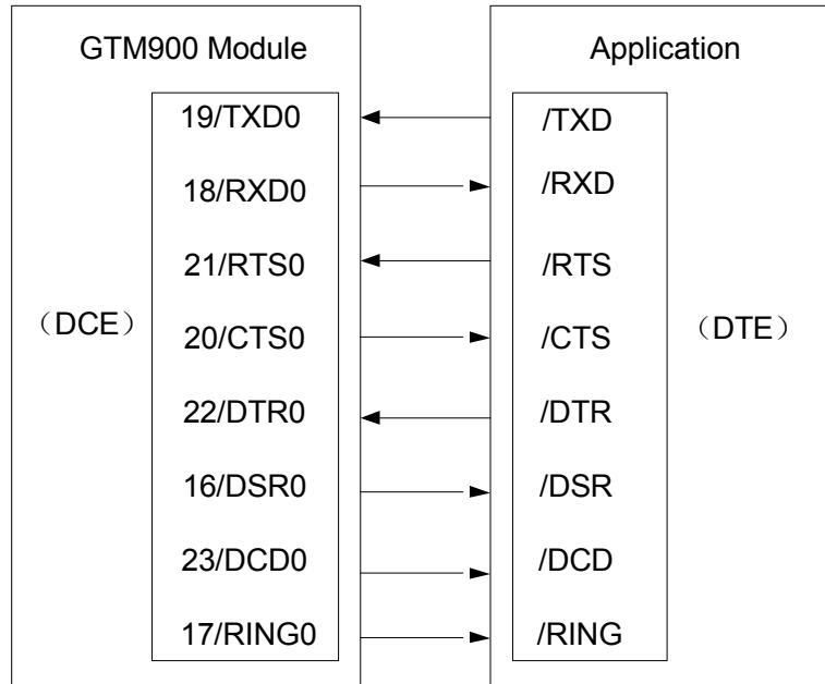
图4-1 DCE-DTE 的连接关系
