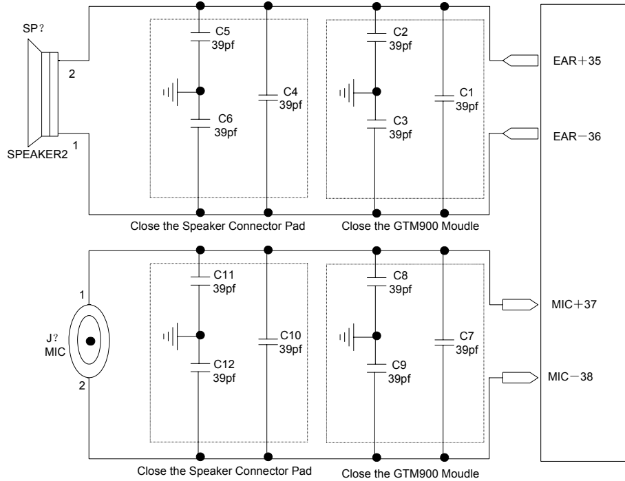
图4-6 第一路音频信号连接示意图
