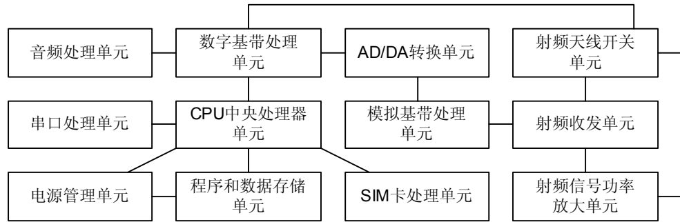
图1-2 逻辑框图
