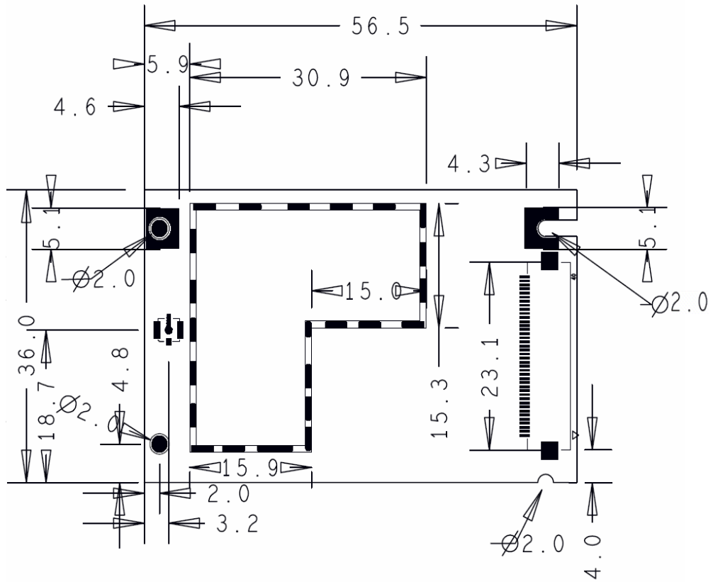
图6-1 结构尺寸图
