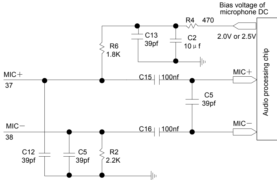
图4-8 第一路音频输入通道的电路示意图
