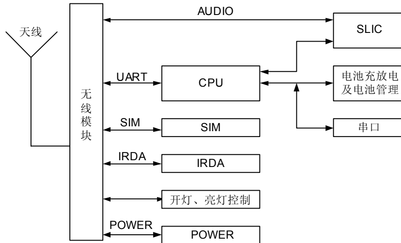
图1-4 Terminal 型逻辑框图
