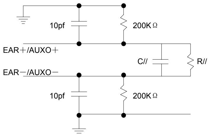
图4-10 音频测试负载电路示意图
