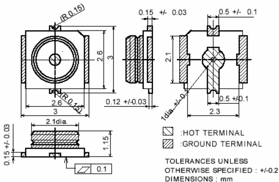
图2-2 天线接口连接器尺寸图（单位：mm）
