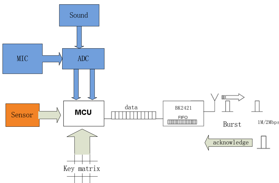
图 6: PC 周边设备 TX 端 (鼠标、键盘、遥控器手写板、MIC、音源.....)
