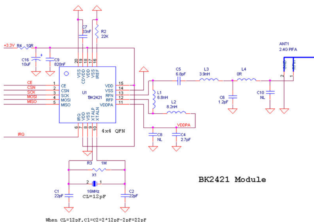
图 10 : BK2421 典型应用电路图
