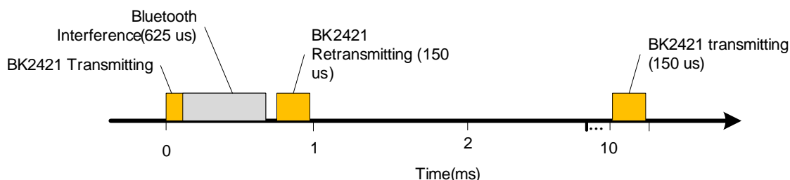
图 3: BK2421 抗 Bluetooth 干扰数据传输图
