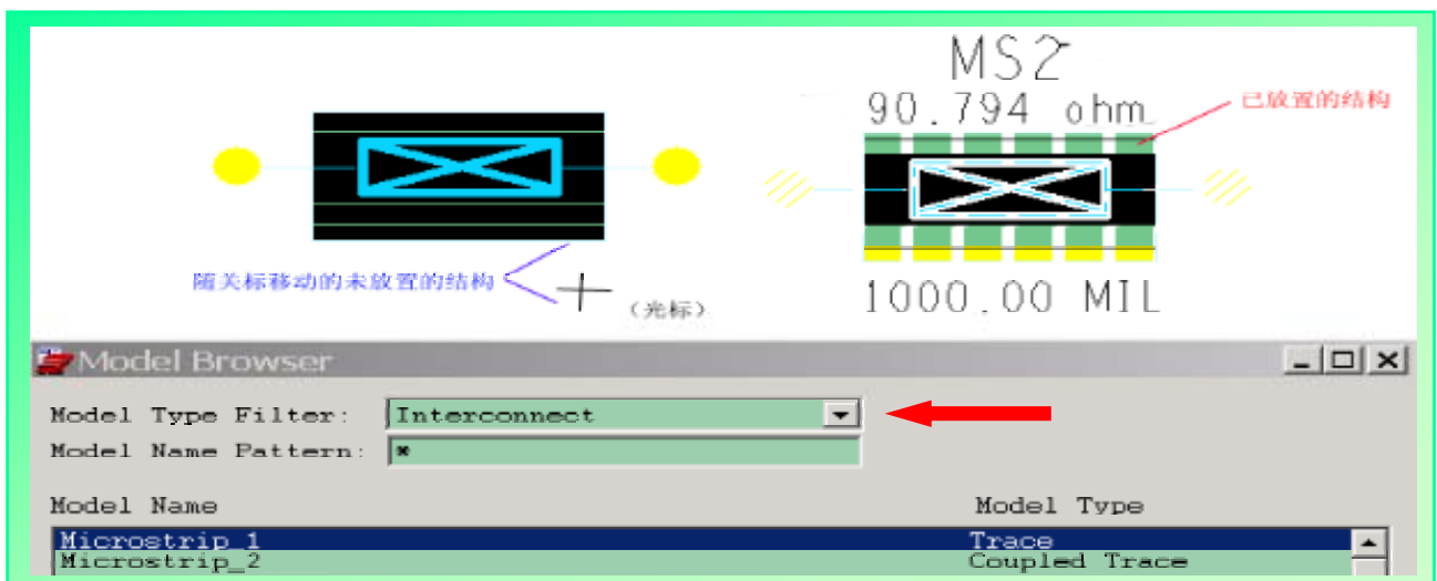
图 8.4 在 Sigplexer 中添加结构体
