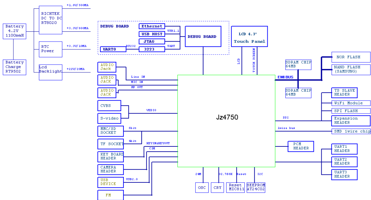
图表 1-1 RD4750_APUS 系统结构图
