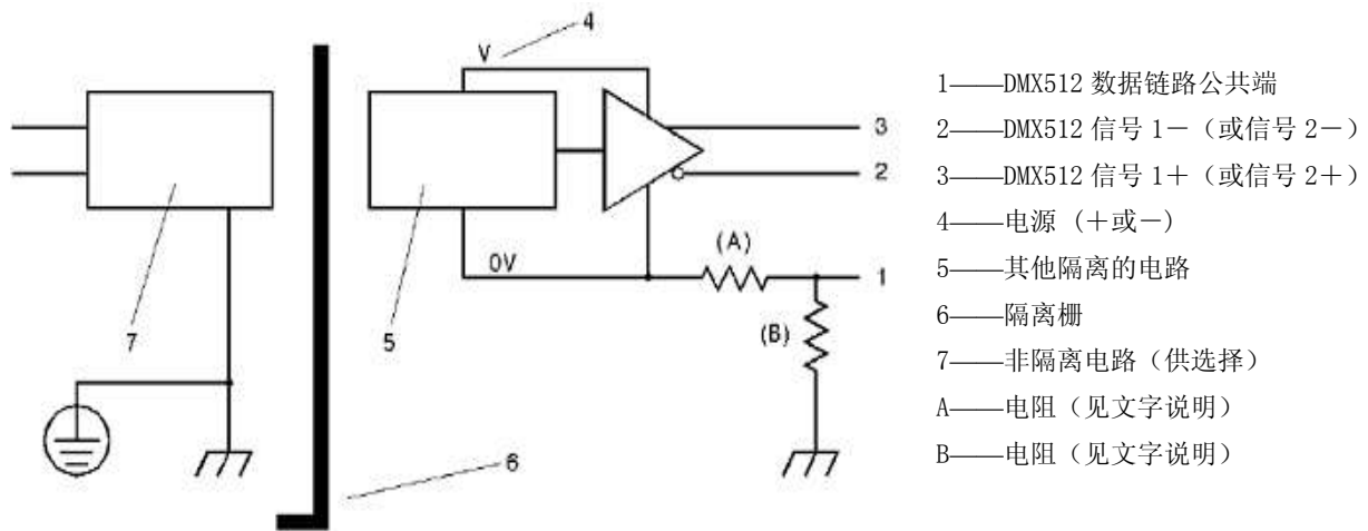
图 A.1 隔离发送器
