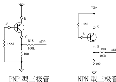
图 33 三极管 hFE 测试
