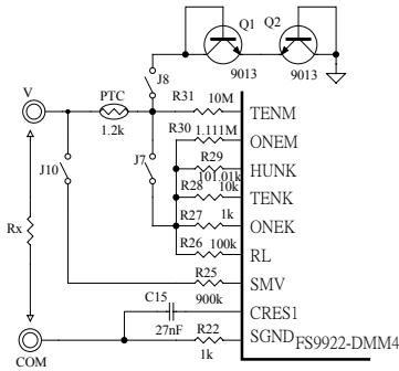
图 30 电阻测量
