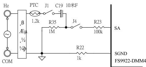
图 36 高频测量
