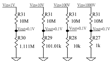
图 26 分压电路示意图
