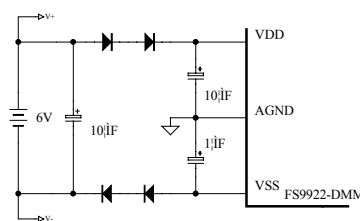
图9 6V 电源供电
