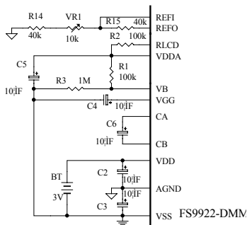
图4 电源电路
