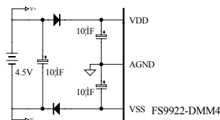
图8 4.5V 电源供电
