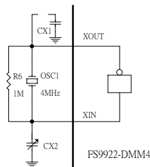
图 16 石英振荡电路
