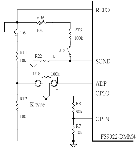
图 39 温度测量 (2)
