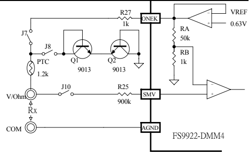
图 32 通断检测
