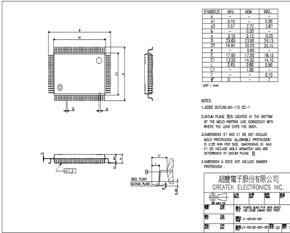
图 42 外观尺寸
