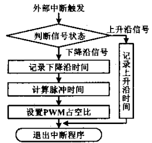
图 6 调速信号检测流程图
