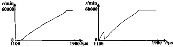
图 8 测试结果
