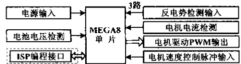
图 3 系统硬件框图
