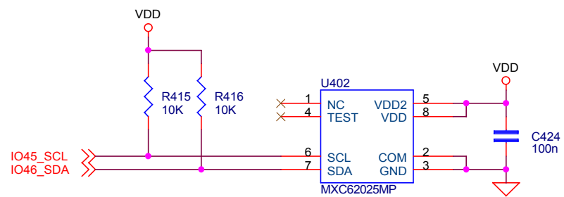
MEMSIC Circuit
